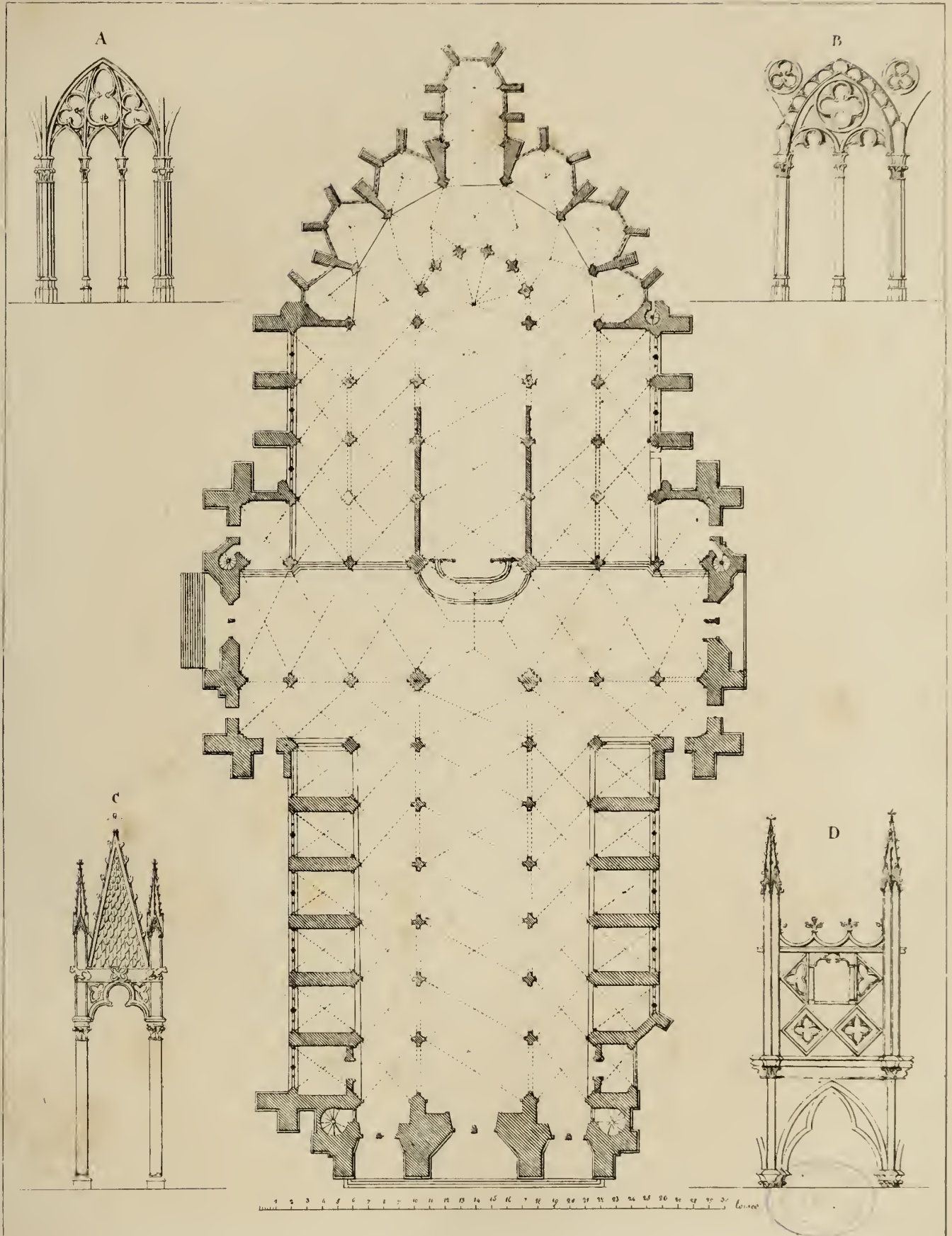
A Arcade de la Galerie Tribune. B Arcade d'une partie antérieure du Porch. C Niche de la Galerie des Rois. D Fragment de la Galerie du Couronnement.
